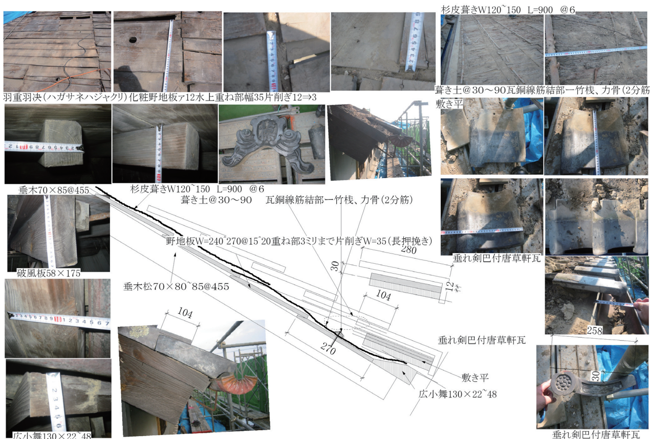
主屋大屋根軒先実測調査図
