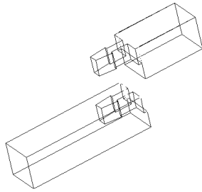
腰掛鎌仕口
