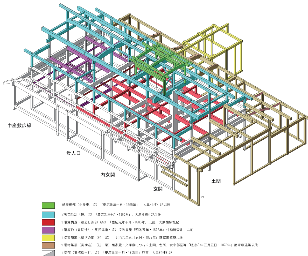
CG・村松家増築、移転前軸組部 南東部鳥瞰図
