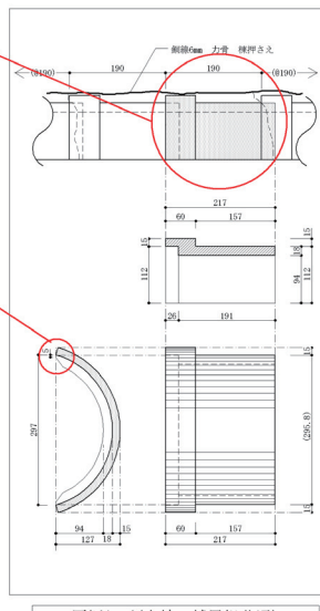
雁振り瓦(大棟、越屋根共通)
