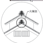
主家 西立面図
