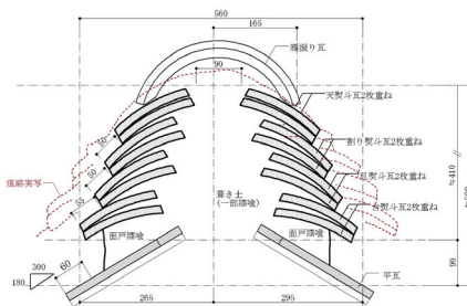
大棟瓦痕跡図(A部)
