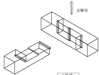
金輪継
