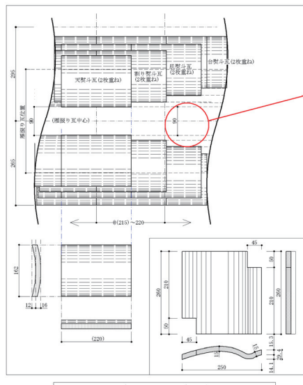
熨斗瓦(大棟、平瓦(大棟、越屋根共通))
